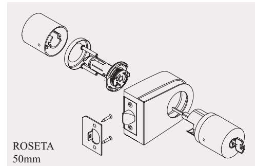
CERROJO
