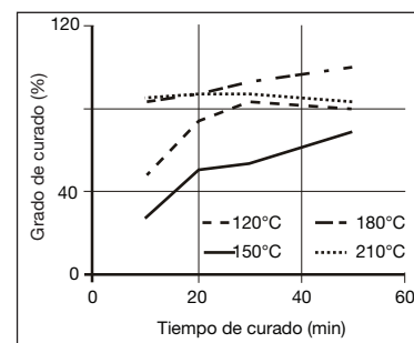
Figura 2: Diagrama de curado (resistencia a cizalladura)
