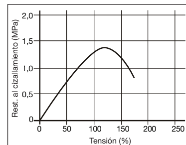
Figura 3: Diagrama de curado (resistencia a cizalladura)
