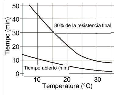
Figura 1: Tiempo abierto y velocidad de curado del SikaFast®-5215
