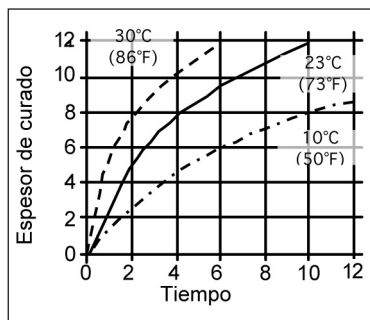
Diagrama 1: Velocidad de curado del Sikaflex®-265 DG-3 (VP)
