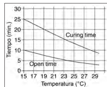
Diagrama 1: tiempo abierto y tiempo de curado para el SikaForce® 7110 L14
