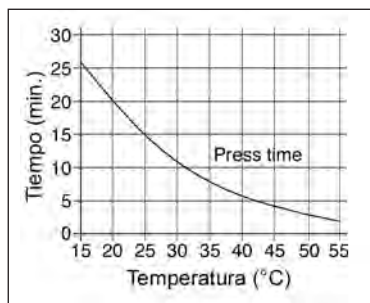
Diagrama 2: tiempo de prensa para el SikaForce® 7110 L14
