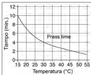
Diagrama 2: tiempo de prensa para el SikaForce® 7110 L5
