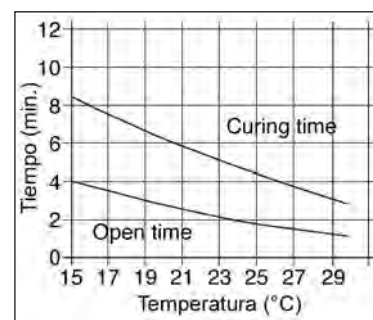
Diagrama 1: tiempo abierto y tiempo de curado para el SikaForce® 7110 L5
