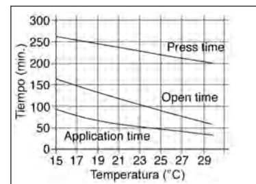
Diagrama 1: tiempo de prensa, tiempo abierto y tiempo de aplicación para el SikaForce® 7710 L100
