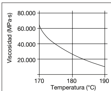
Diagrama 1: Viscosidad del SikaMelt®-9285 en función de la temperatura.
