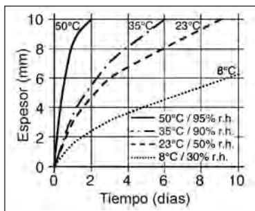
Diagrama 1: Velocidad de curado del SikaSil WT 40.
