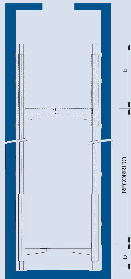
ALZADO
