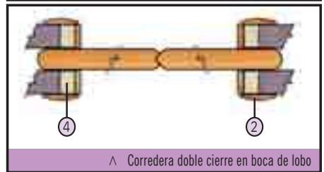
^ Corredera solapada
