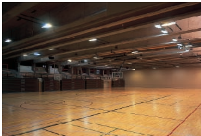
Las altas prestaciones fotométricas del FR 42 y del FR 44 permiten reducir el número de proyectores a instalar.
