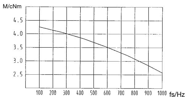
UOJ5 (ST 5022/11,25/1)
