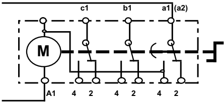
KKH--388
