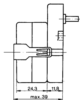
UDR 1..A
