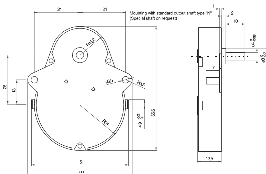
UDS 1..D
