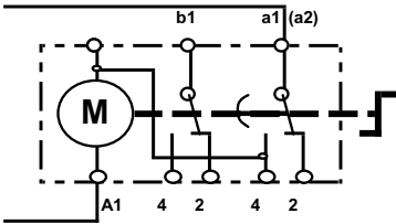
KKH--288
