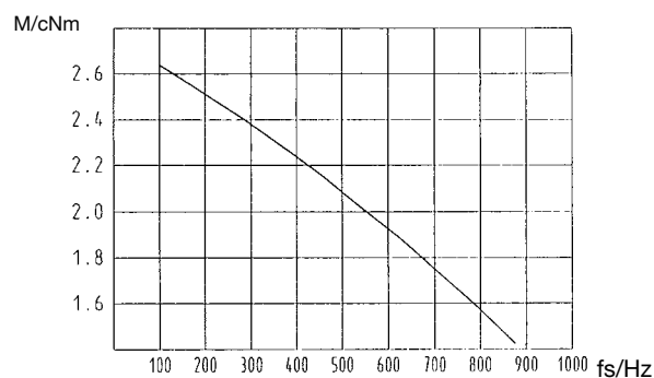
UOJ5 (ST 5022/11,25/1)
