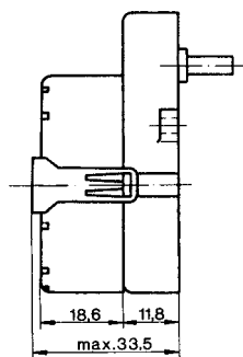
UDS 1..A
