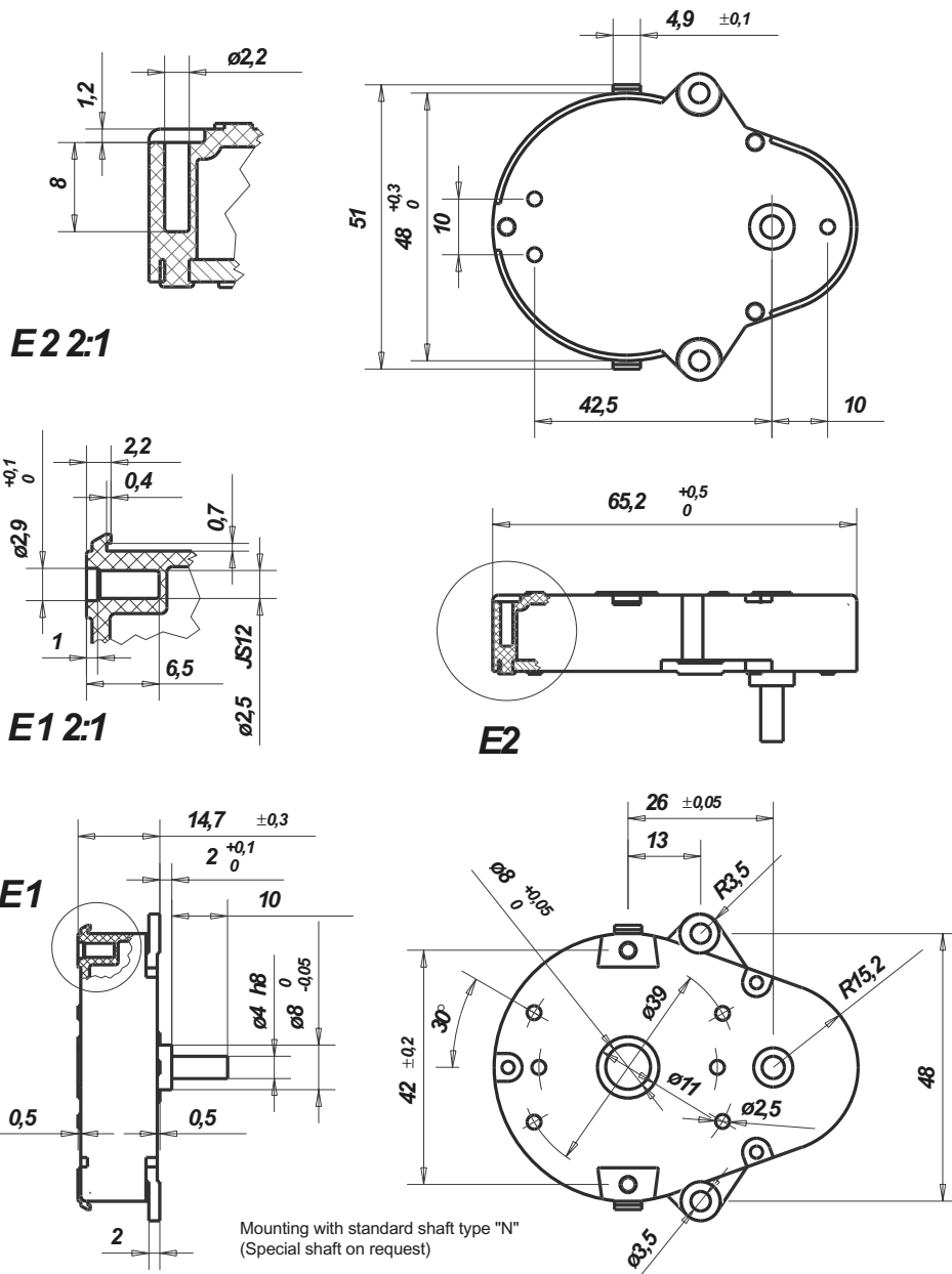
UDS 1..M
