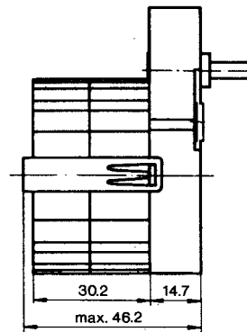
UFR 1..M
