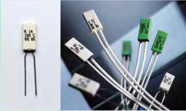
Tipo O (n.a.) y P (n.c.), rearme aut. Tipo Q con R mantenimiento tipo PTC 40-150°C, 230Vac-5(3.2)A, VDE/UL
