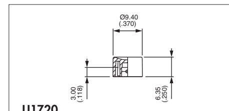
U1720
