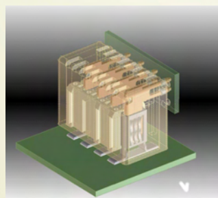
Adaptador 1,27 mm
