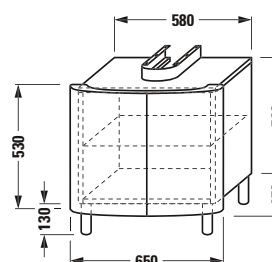
4.6194.2.994.YYY.1 Base mueble para lavabo, frontal bajo, 2 puertas, 1 estante vidrio, 4 pies.
