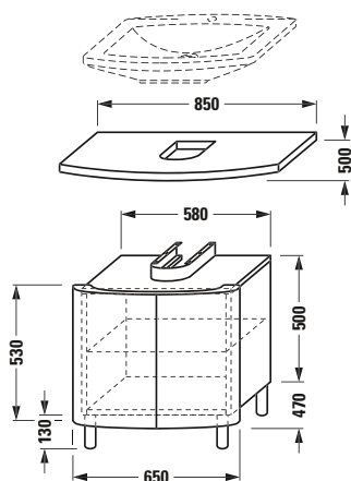
4.6194.5.994.YYY.1 Base mueble con encimera para lavabo 8.1894.4.000.XXX.1, frontal bajo, 2 puertas, 1 estante vidrio, 4 pies
