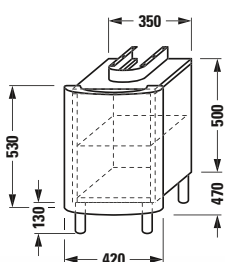
4.4202.1.994.YYY.1* Base mueble para lavabo, frontal bajo, 4.4202.2.994.YYY.1* 1 puerta, 1 estante vidrio, 4 pies.
