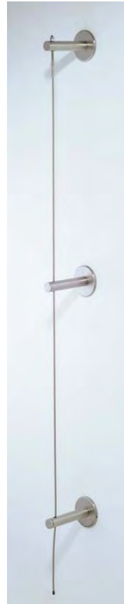
Edelstahlseil 4 mm, 820-0400 einseitig Außengewinde verpresst 850-0400-060 anderseitig Seilende glatt mit Seilendkappe 904-0400 Stainless steel wire rope 4 mm, 820-0400 one side external thread swaged 850-0400-060 other side wire rope end cap 904-0400
