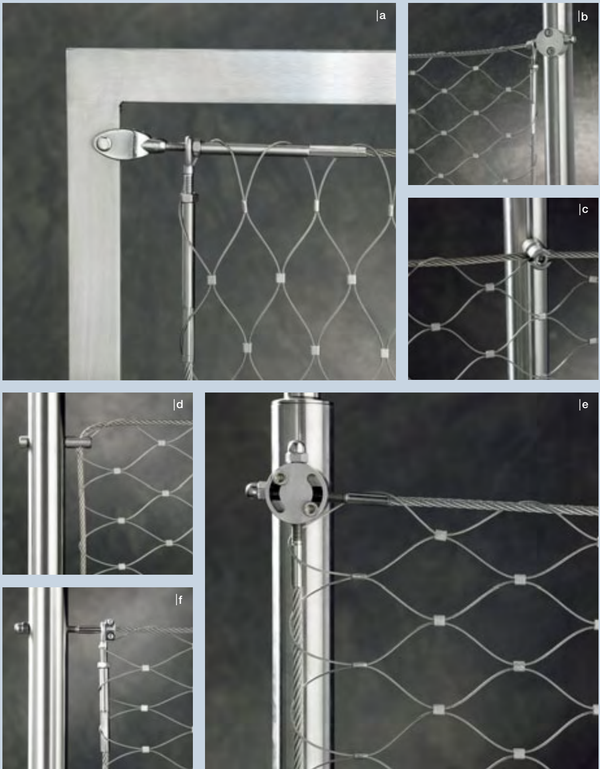
a-f Randseile und Befestigungen | Border cables and fixing points | Câbles de périphérie et fixations
