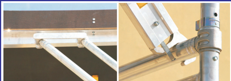
Enganche de última barandilla y de escalera interior
