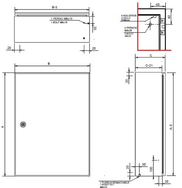
Plano Genérico
