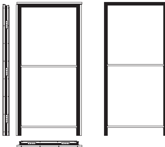
Armazón revoque
